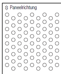
∅ 1,5 mm ⇄ 3 ⇄ 5,2 Freier Querschn. 23%
