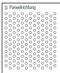
∅ 1 mm ⇄ 2 ⇄ 3,46 Freier Querschn. 23%
