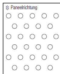
∅ 2 mm ⇄ 8,66 ⇄ 5 Freier Querschn. 16%
