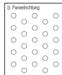
∅ 2* mm ⇄ 5 ⇄ 8,66 Freier Querschn. 16%
